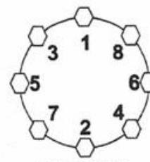
8-Lug Nuts
